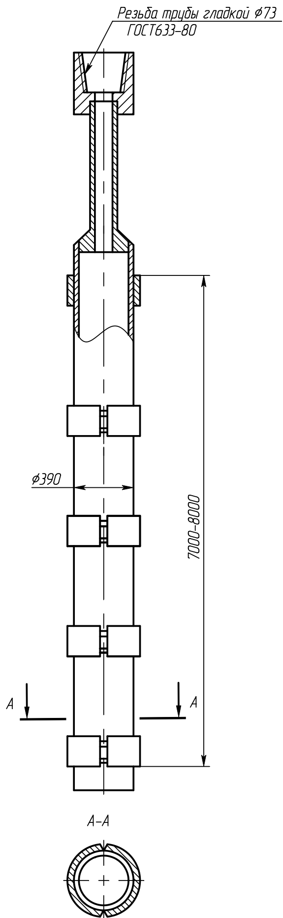
Рис. 3 Шаблон специальный
