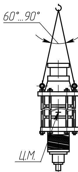
Схема строповки
